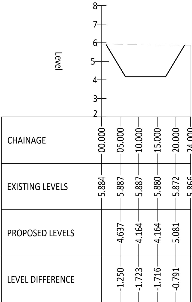
BASIN 3 SECTION F-F SCALE: H 1:500,V 1:100. DATUM: 2.000
