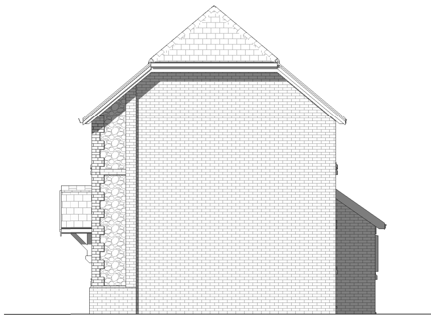
6 Side Elevation - Right G3 1 : 100
