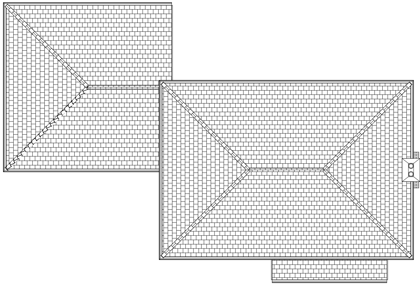
8 0.03 Roof Plan 1 : 100
