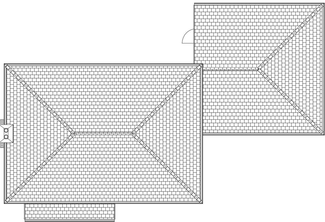
8 0.02 Roof Plan 1 : 100
