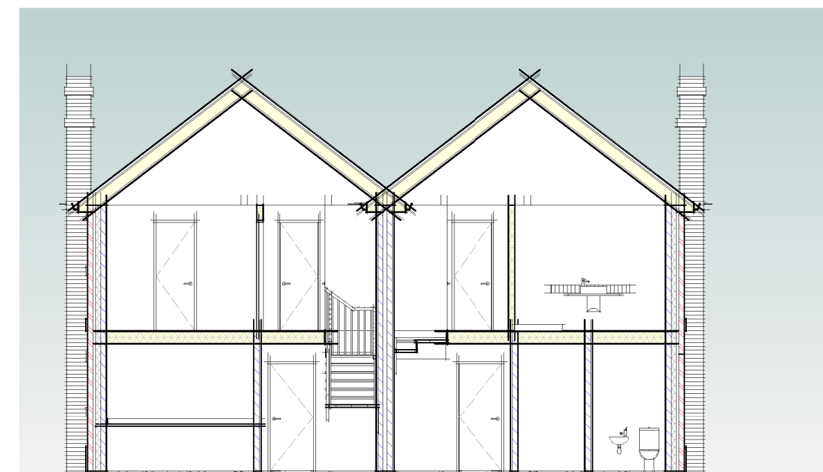
Section 1 1 : 100
