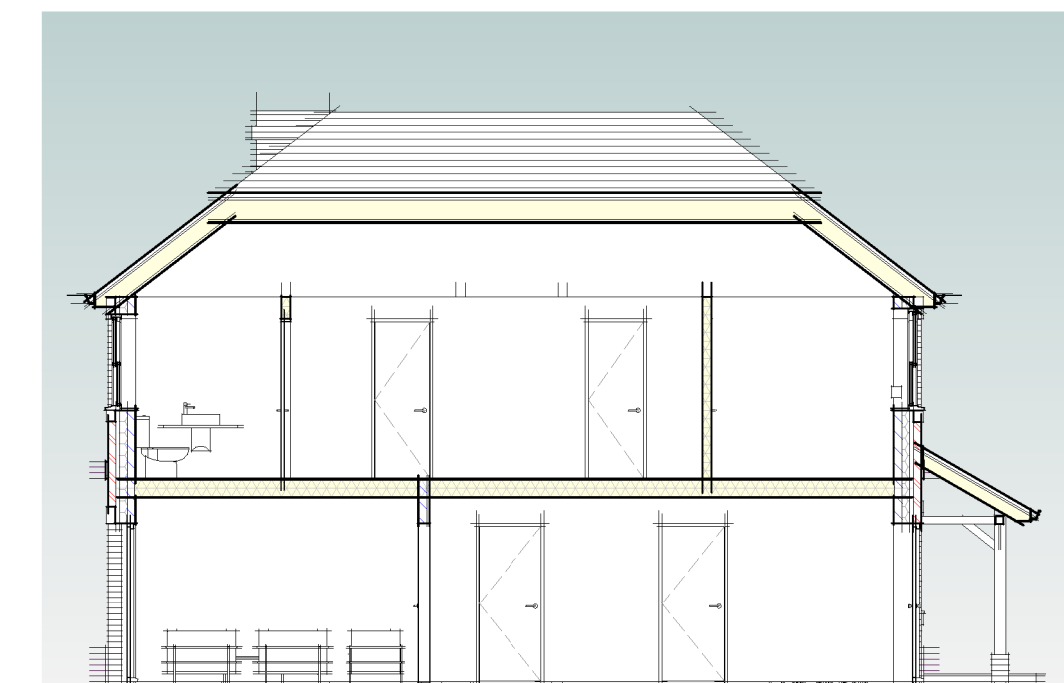
Section 2 1 : 100
