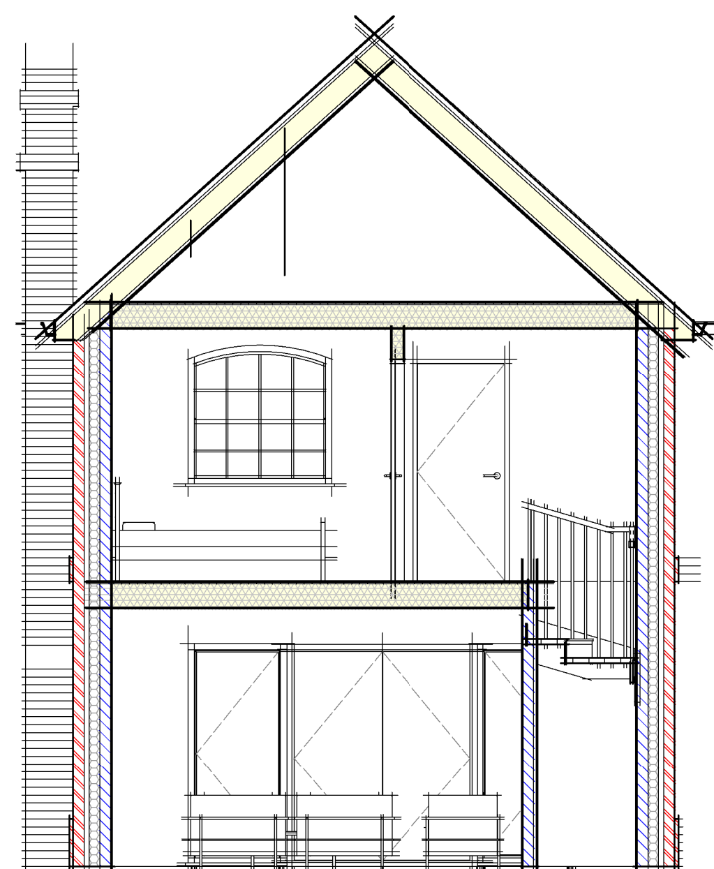
Section 1 1 : 50
