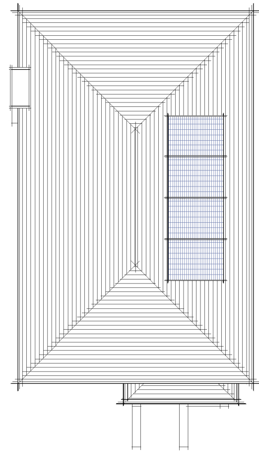
Roof Plan 1 : 100
