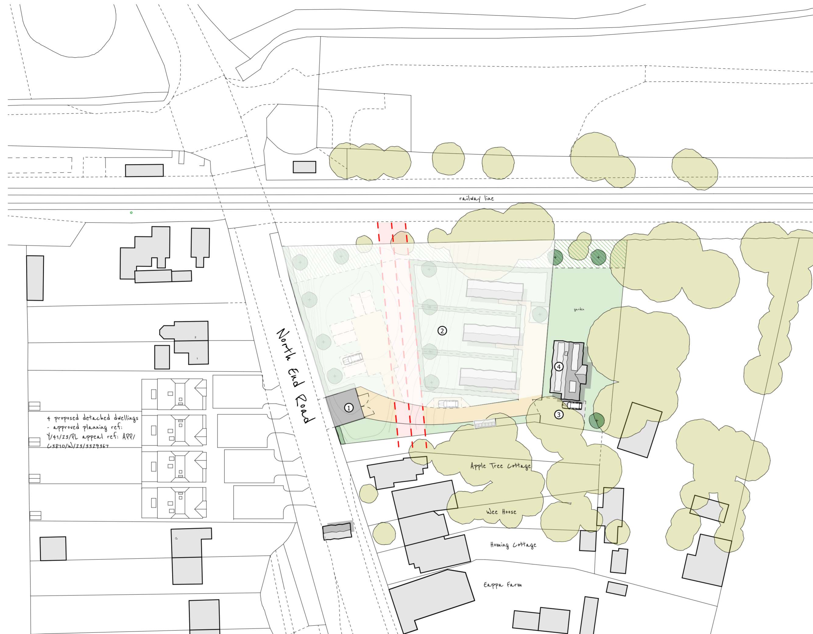
SITE PLAN 1:500
