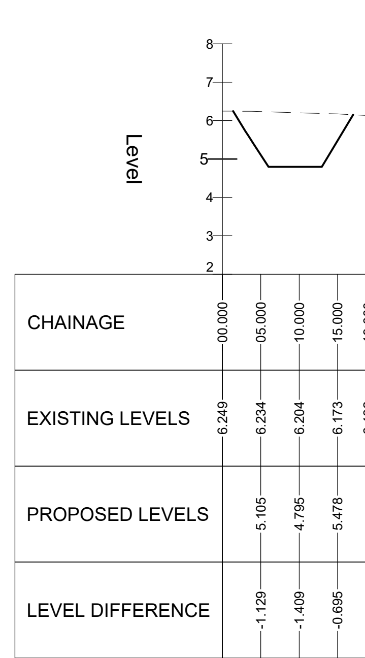
BASIN 2 SECTION D-D SCALE: H 1:500,V 1:100. DATUM: 2.000
