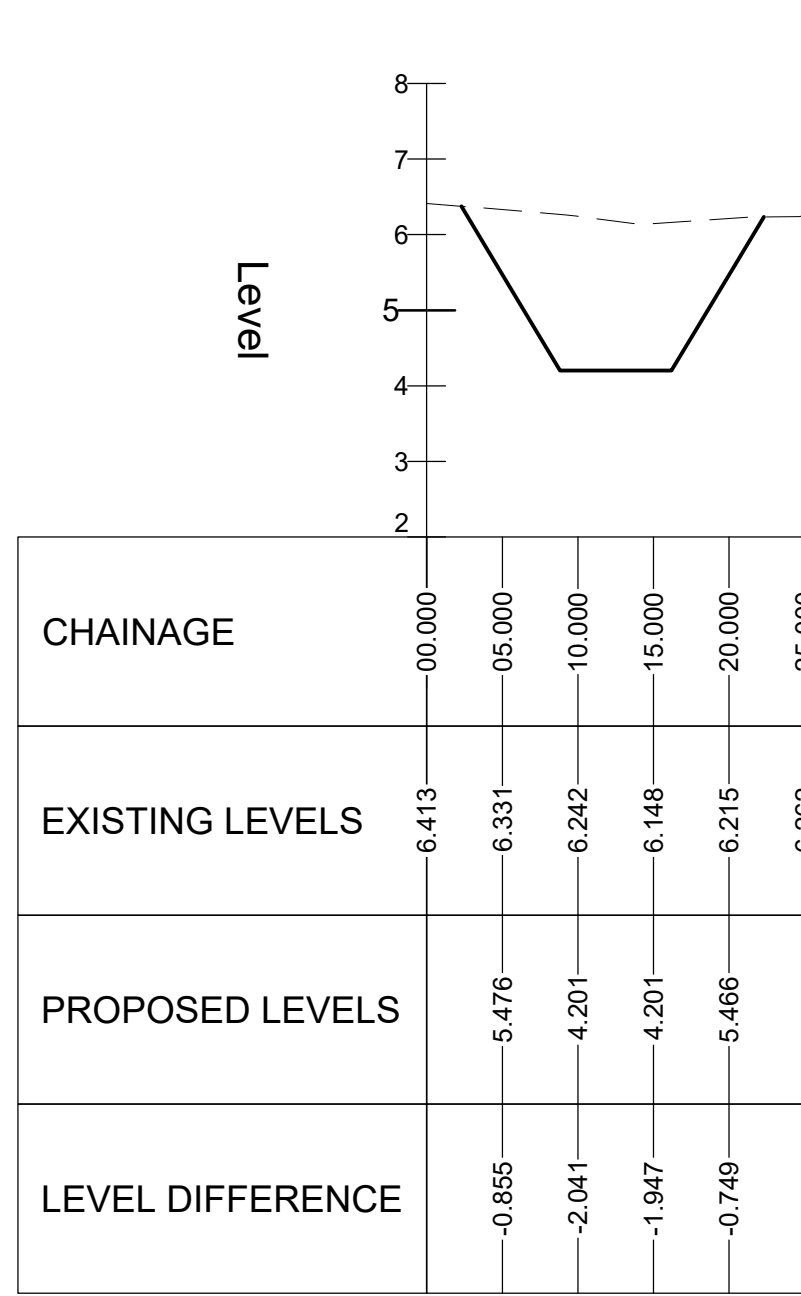
BASIN 1 SECTION B-B SCALE: H 1:500,V 1:100. DATUM: 2.000
