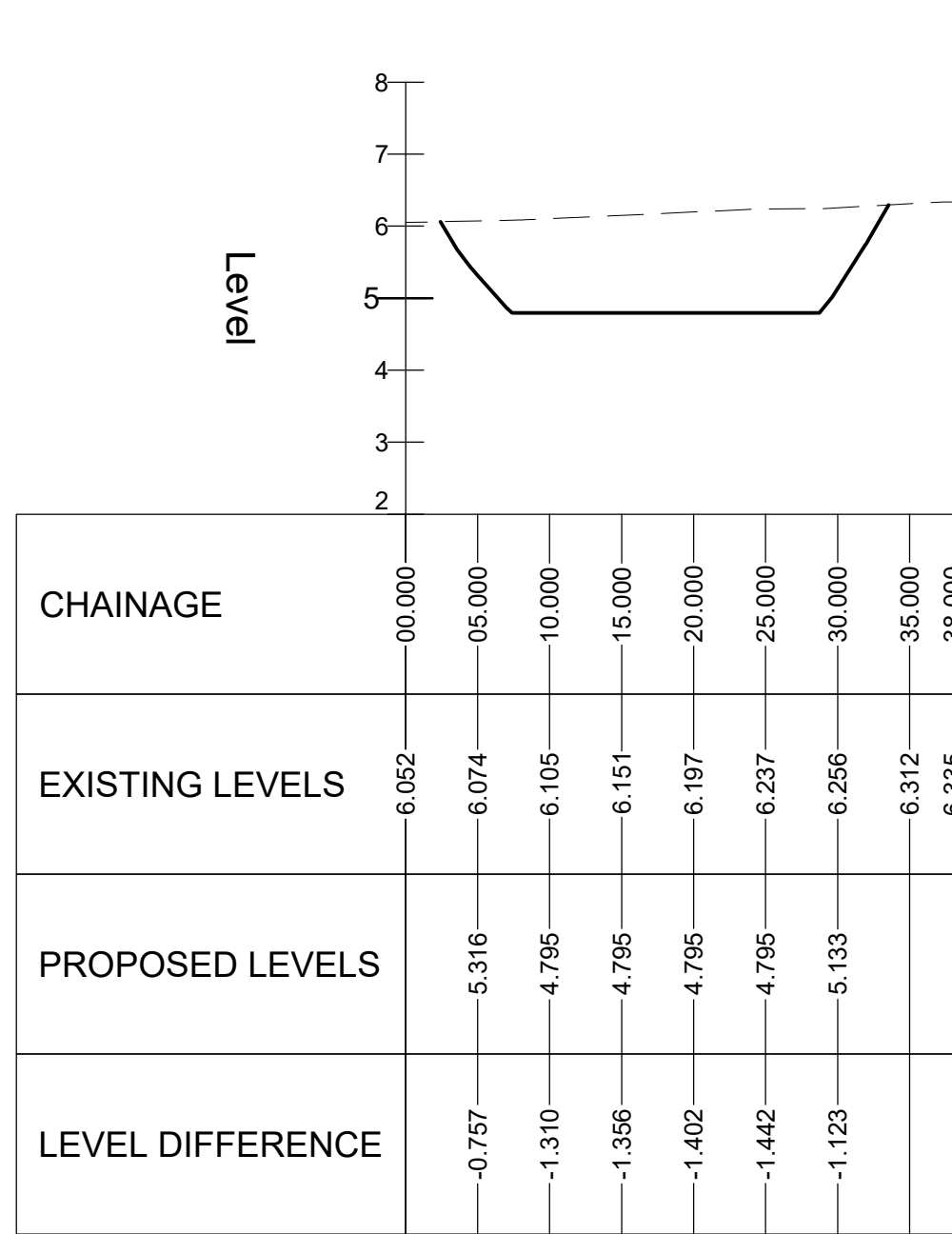
BASIN 2 SECTION C-C SCALE: H 1:500,V 1:100. DATUM: 2.000
