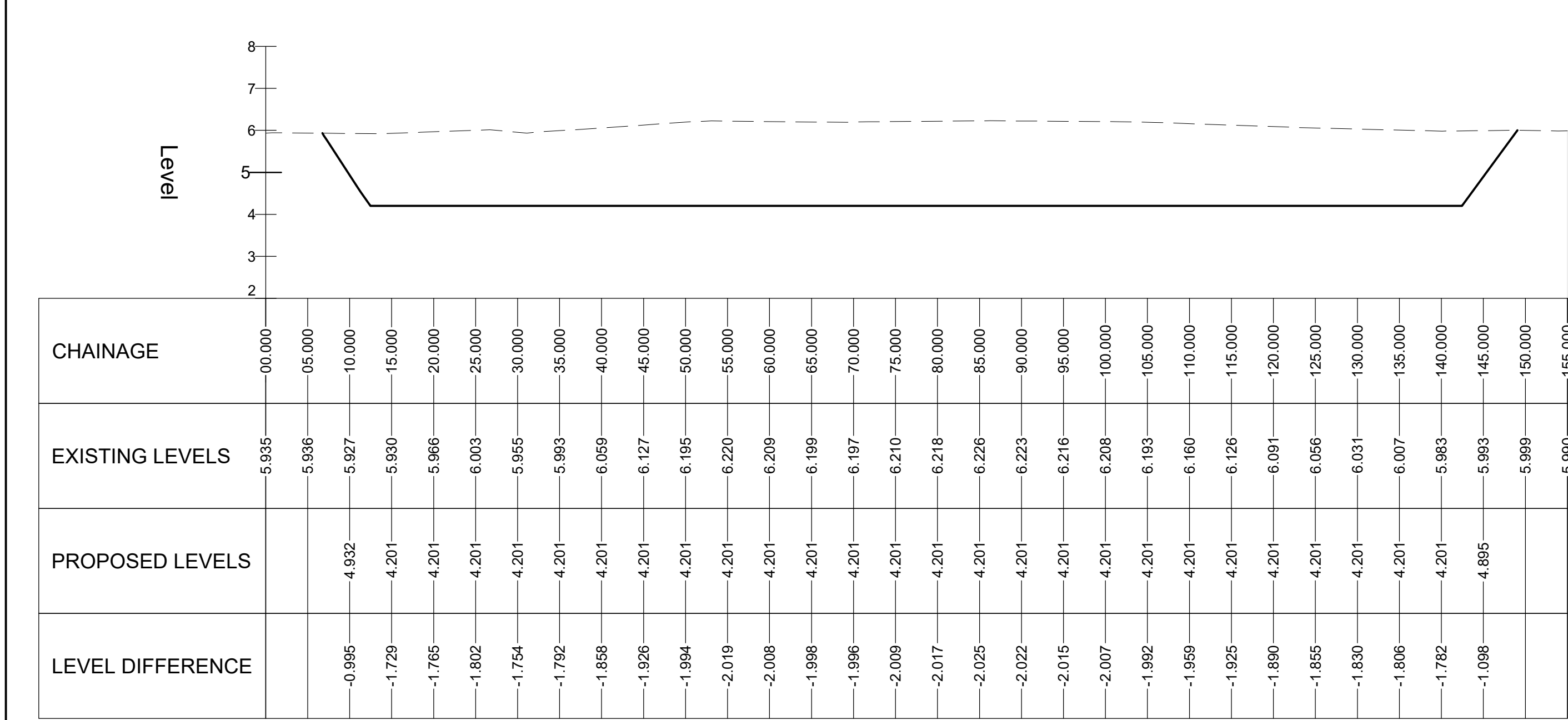
BASIN 1 SECTION A-A SCALE: H 1:500,V 1:100. DATUM: 2.000
