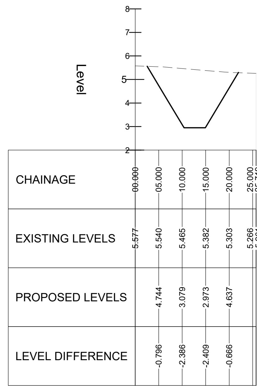
BASIN 5 SECTION K-K SCALE: H 1:500,V 1:100. DATUM: 2.000
