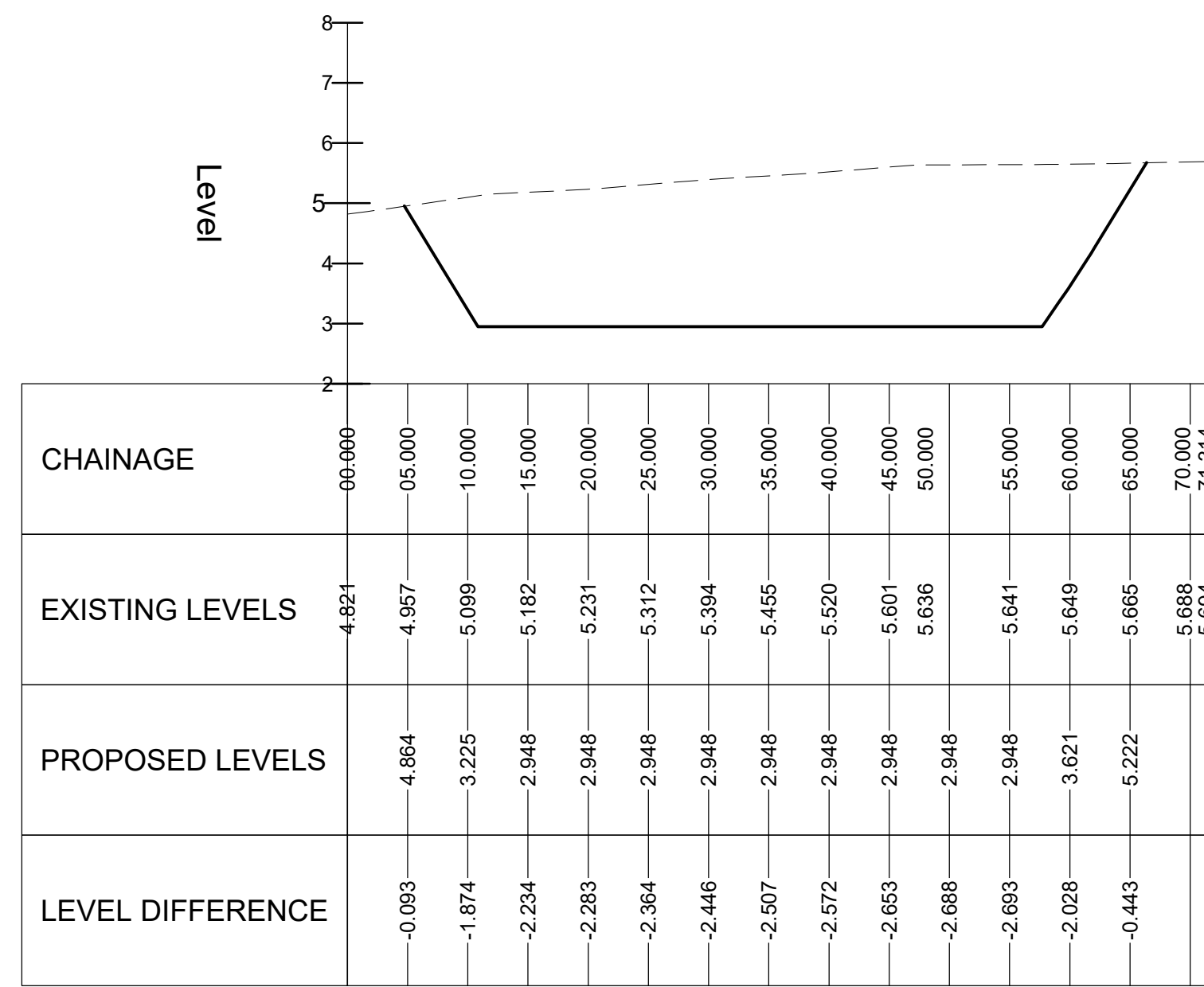
BASIN 5 SECTION J-J SCALE: H 1:500,V 1:100. DATUM: 2.000
