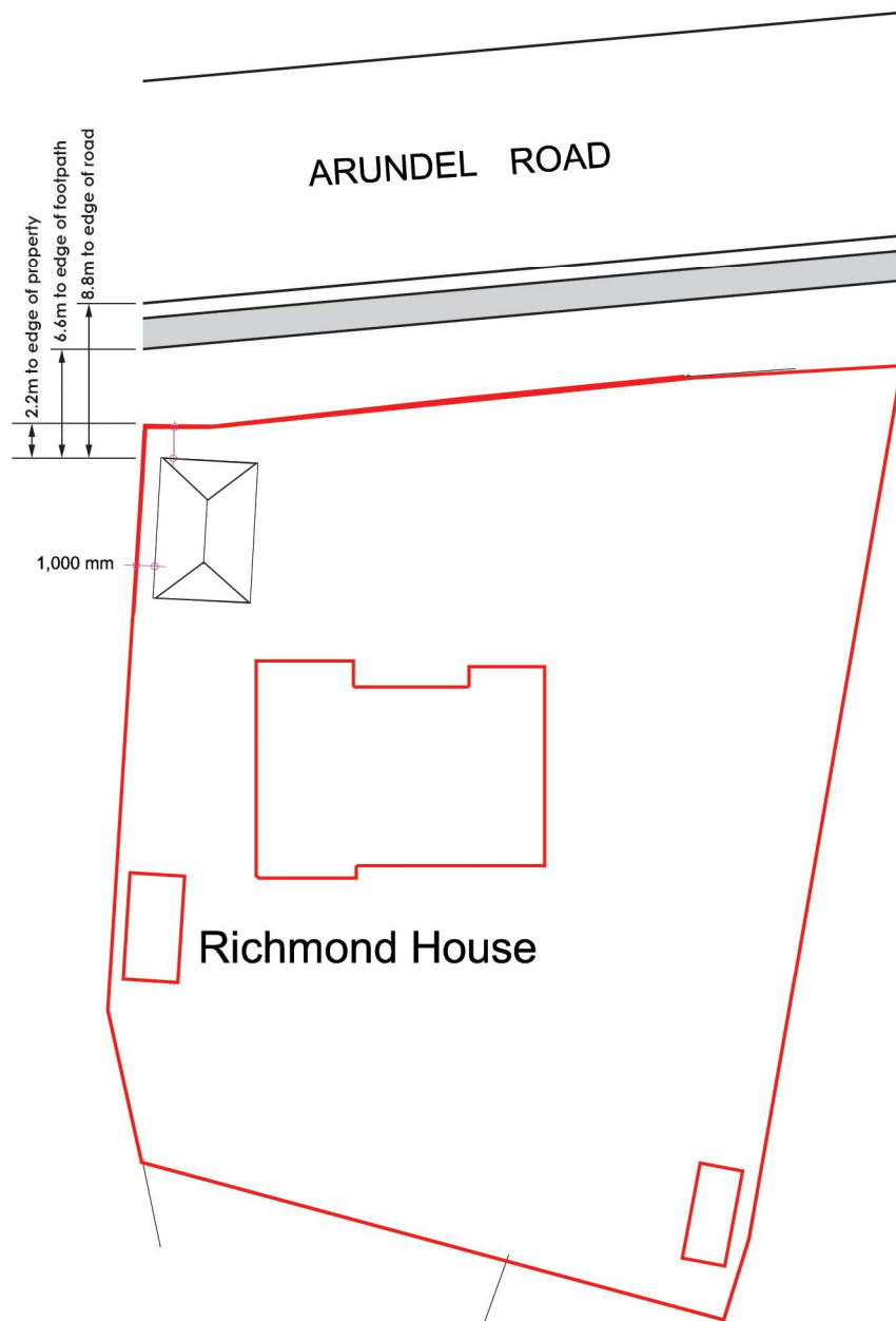
SITE PLAN - 1/500
