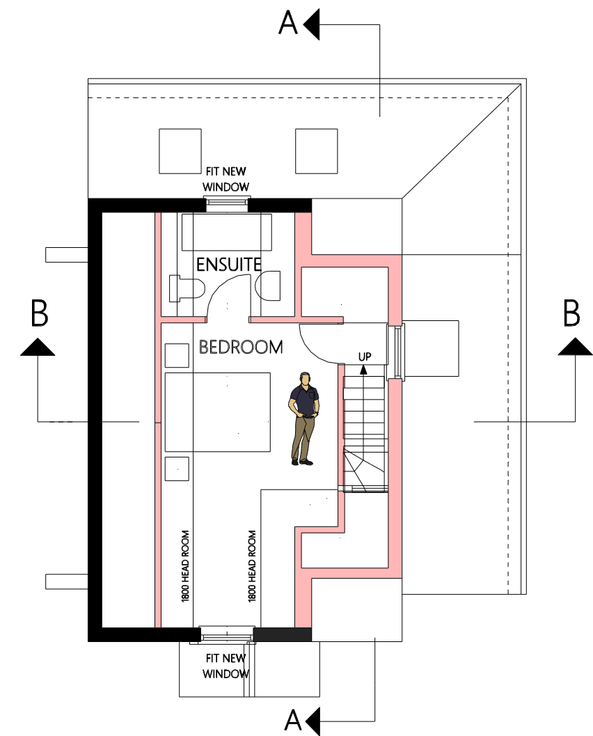
LOFT PLAN
