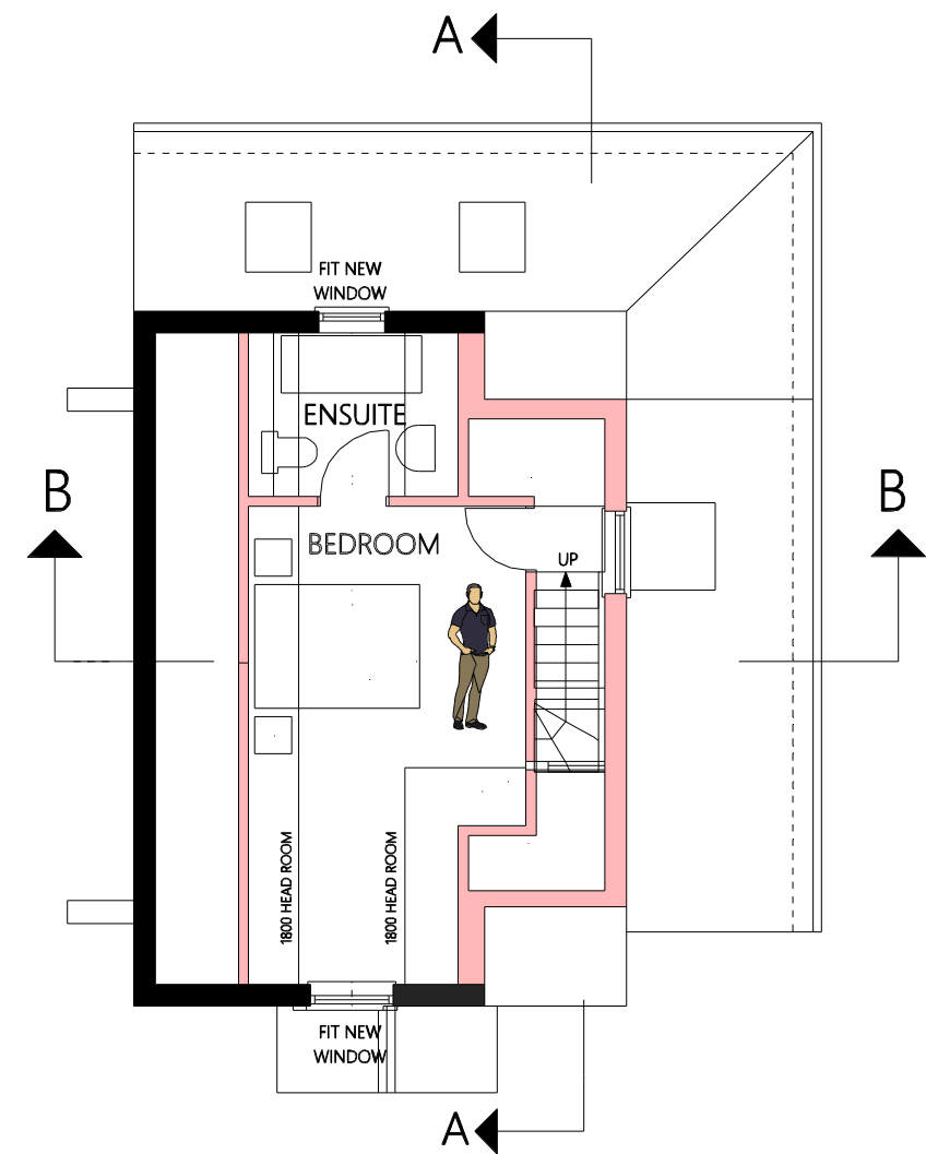
LOFT PLAN
