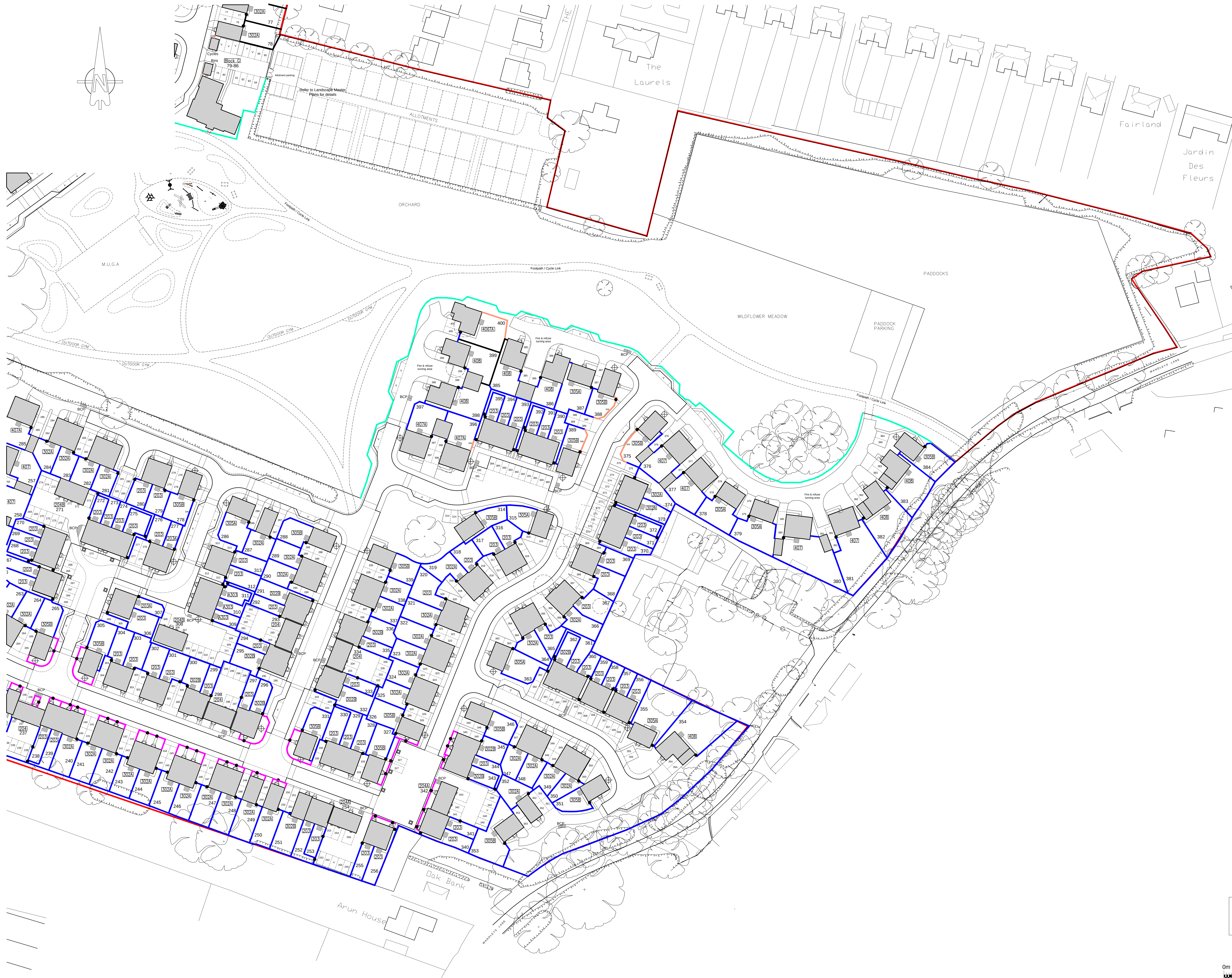
SITE LAYOUT 1:500
