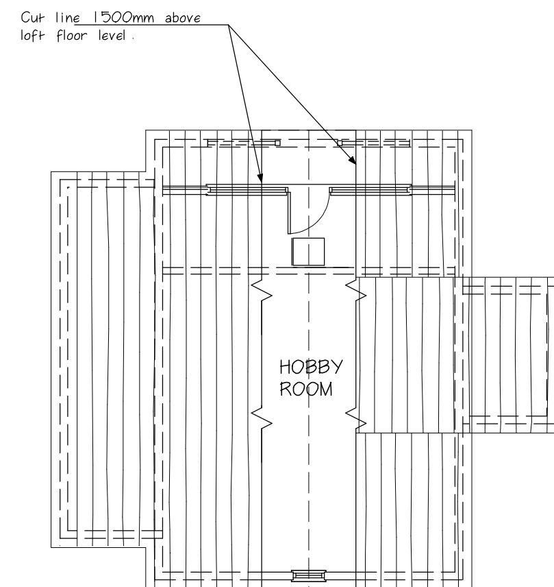
LOFT PLAN 1:100
