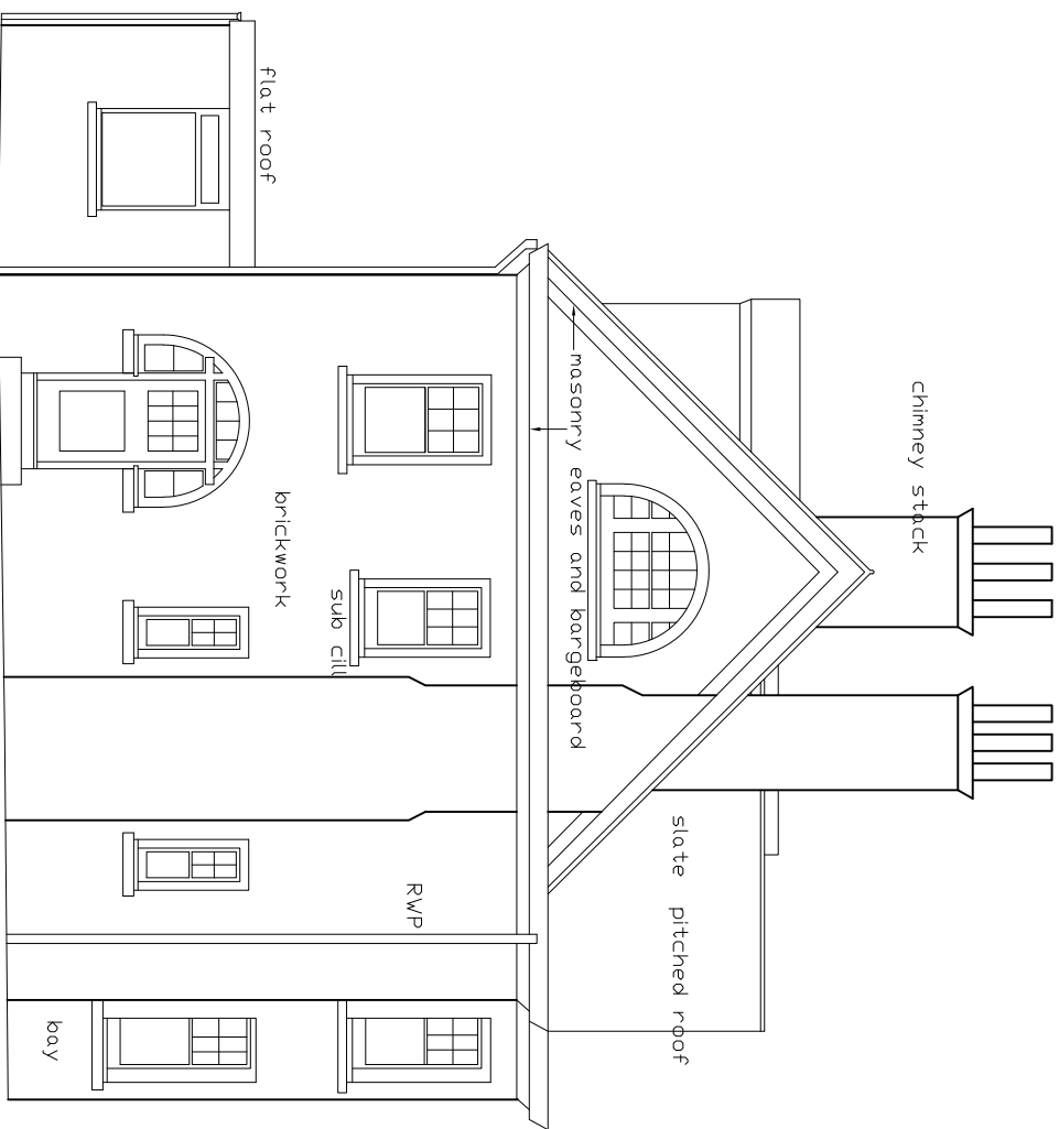
WEST ELEVATION Scale: 1:100
