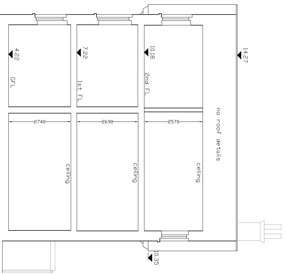
SECTION 2-2 Scale: 1:100
