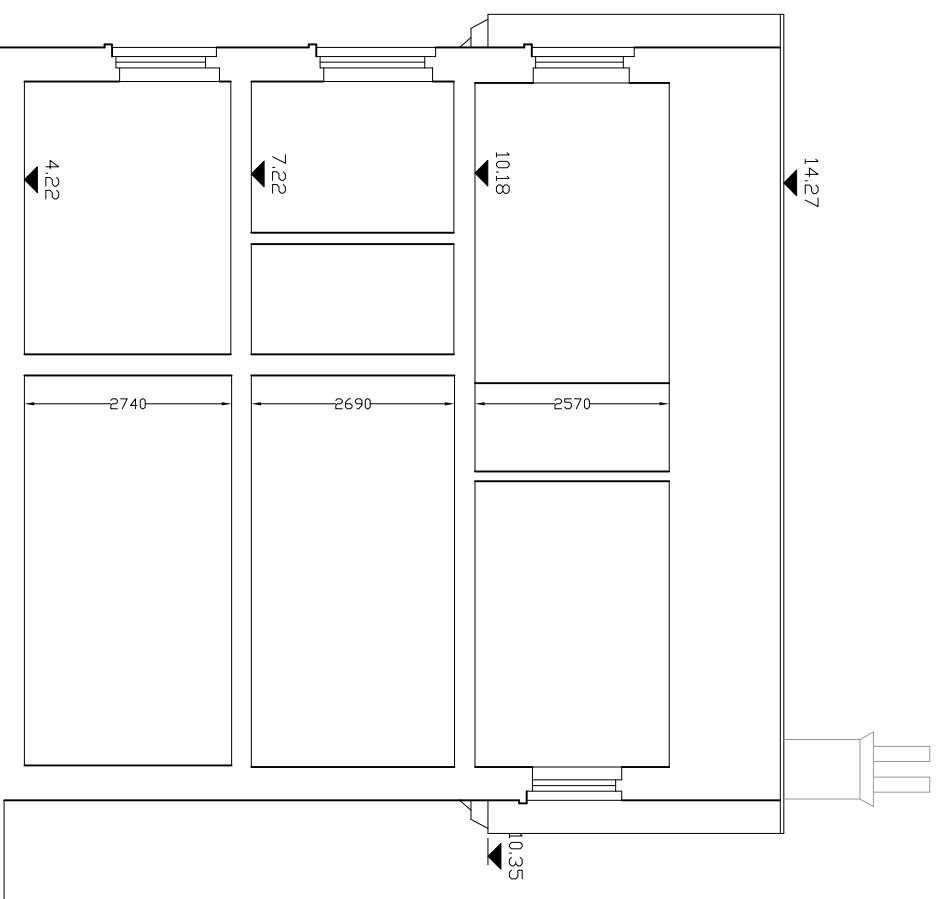
SECTION 2 Scale: 1 : 100
