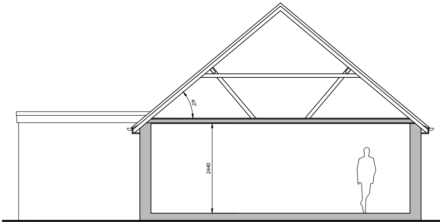
SECTION 1:100 @ A3
