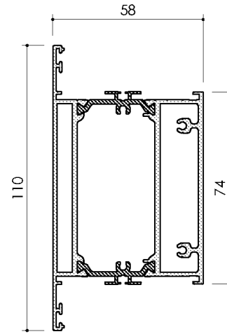
588W ST / AW435
