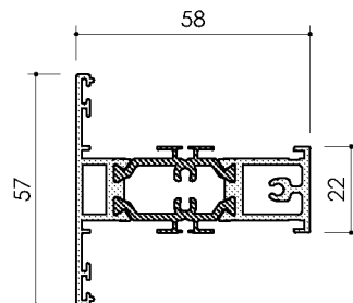
588W ST / AW432
