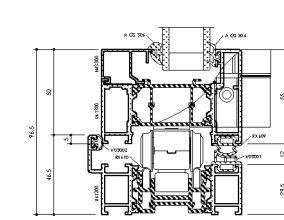
F82 Cill
