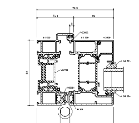
F82 Jamb
