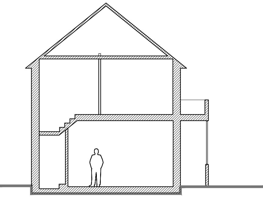
Section A-A 1:100
