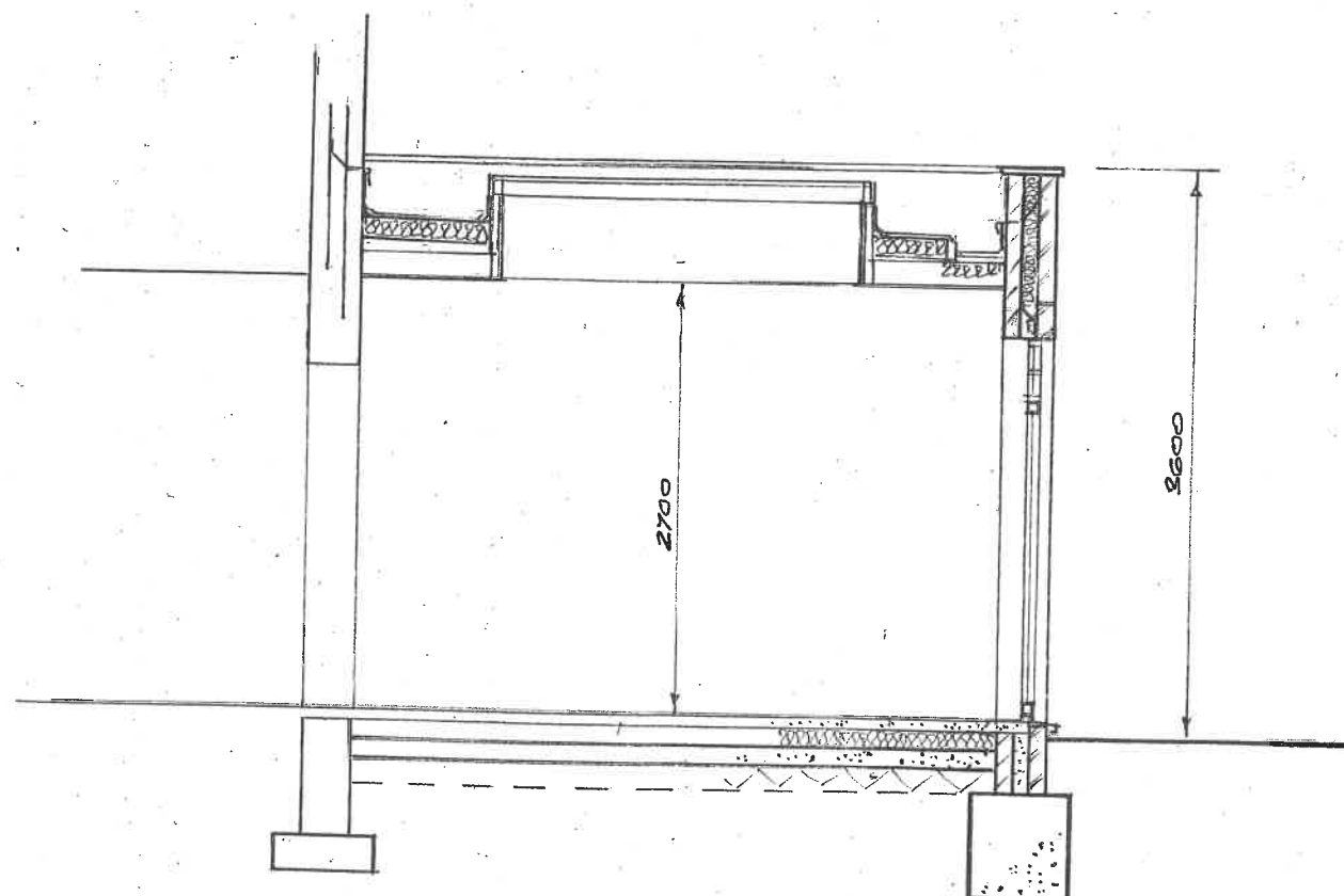
SECTION A-A
