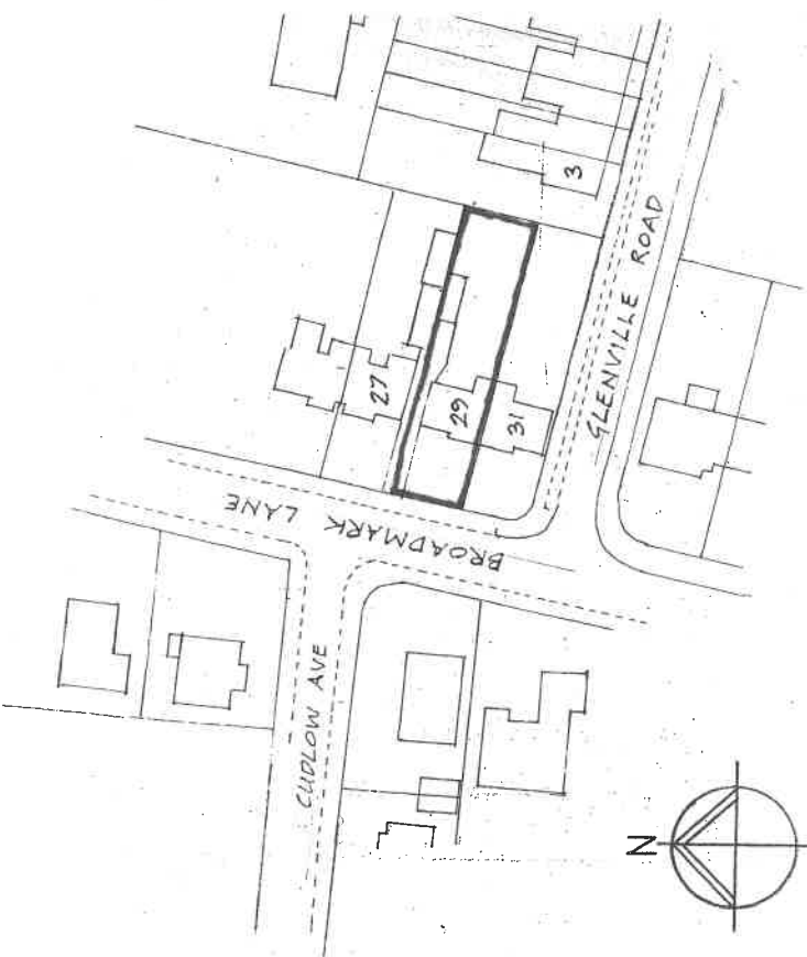
SITE PLAN 1:1250
