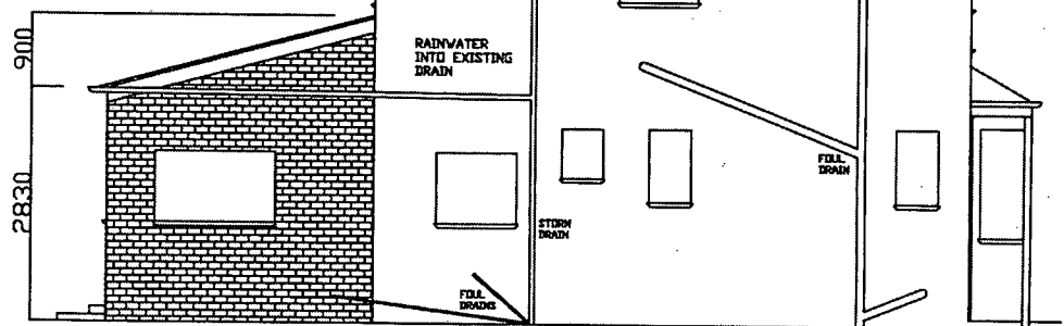
Flank Elevation
