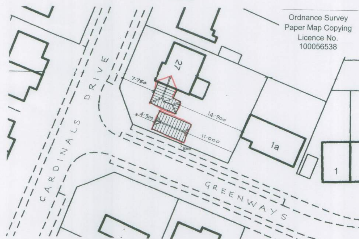
block plan 1 : 500
