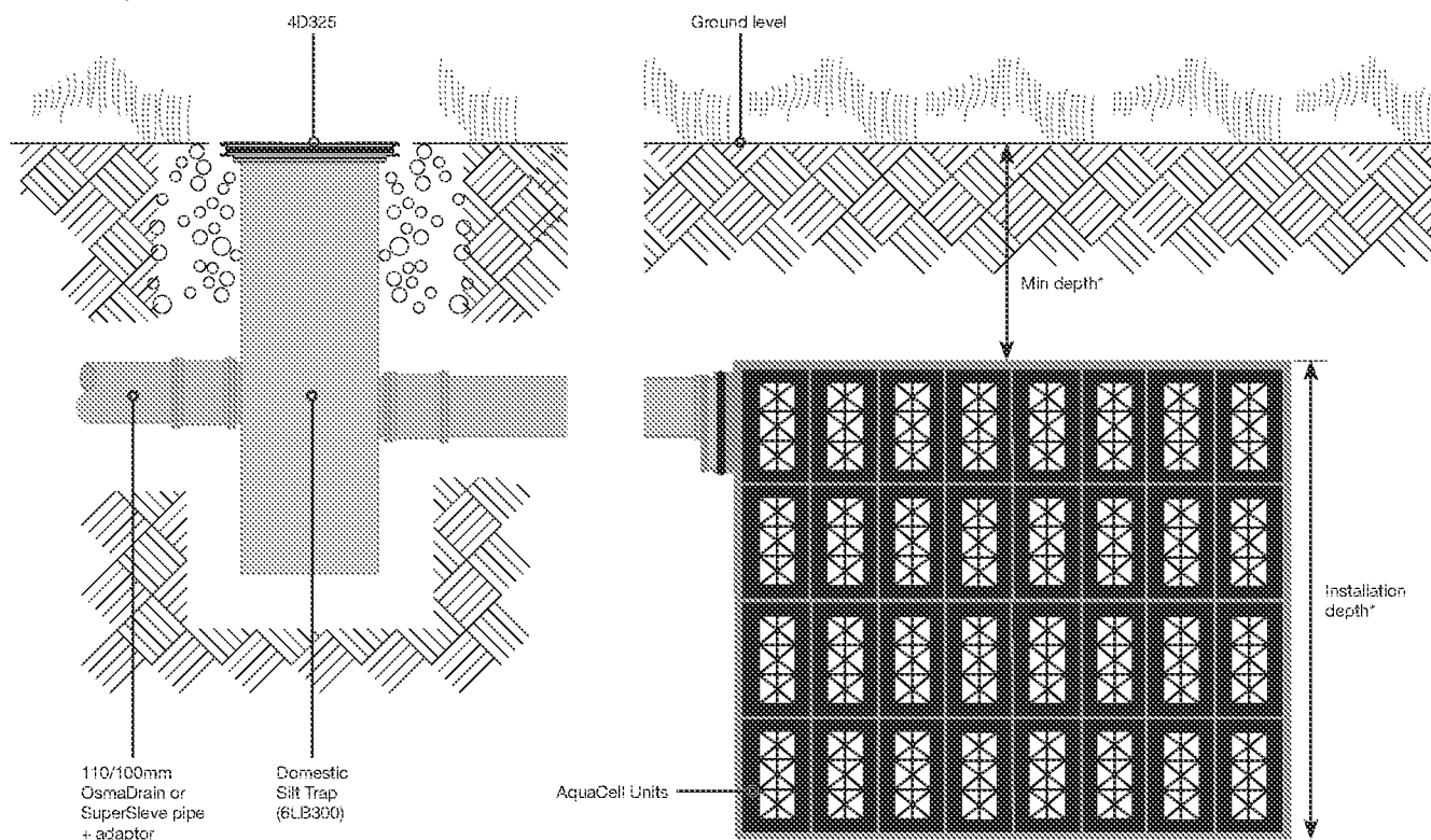
Soakaway
