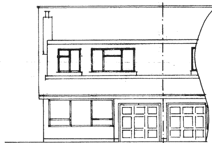
front 1 : 100
