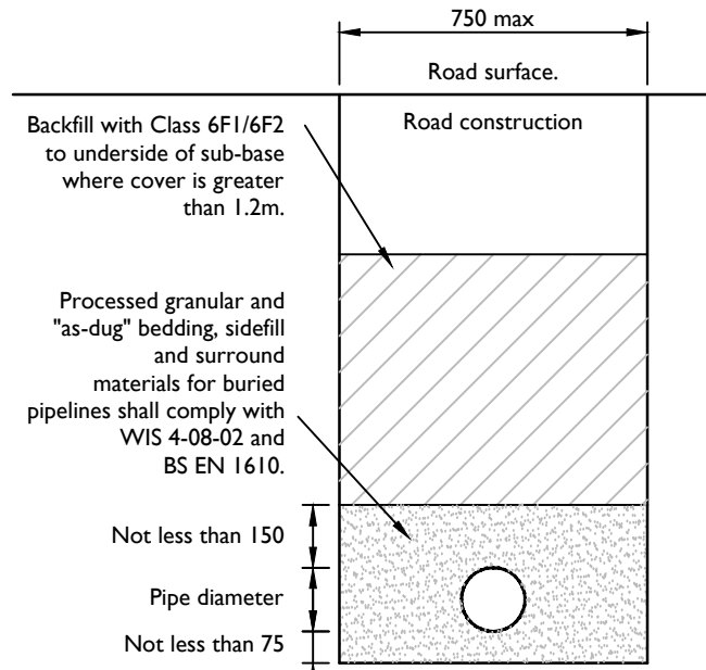
RIISING MAIN PIPE BEDDING DETAIL (Scale 1:20)
