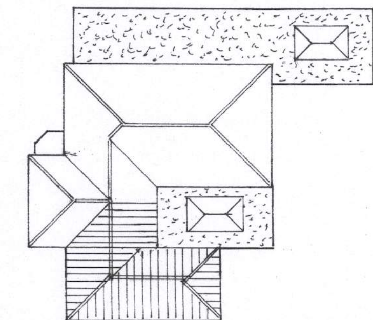
roof plan 1 : 200
