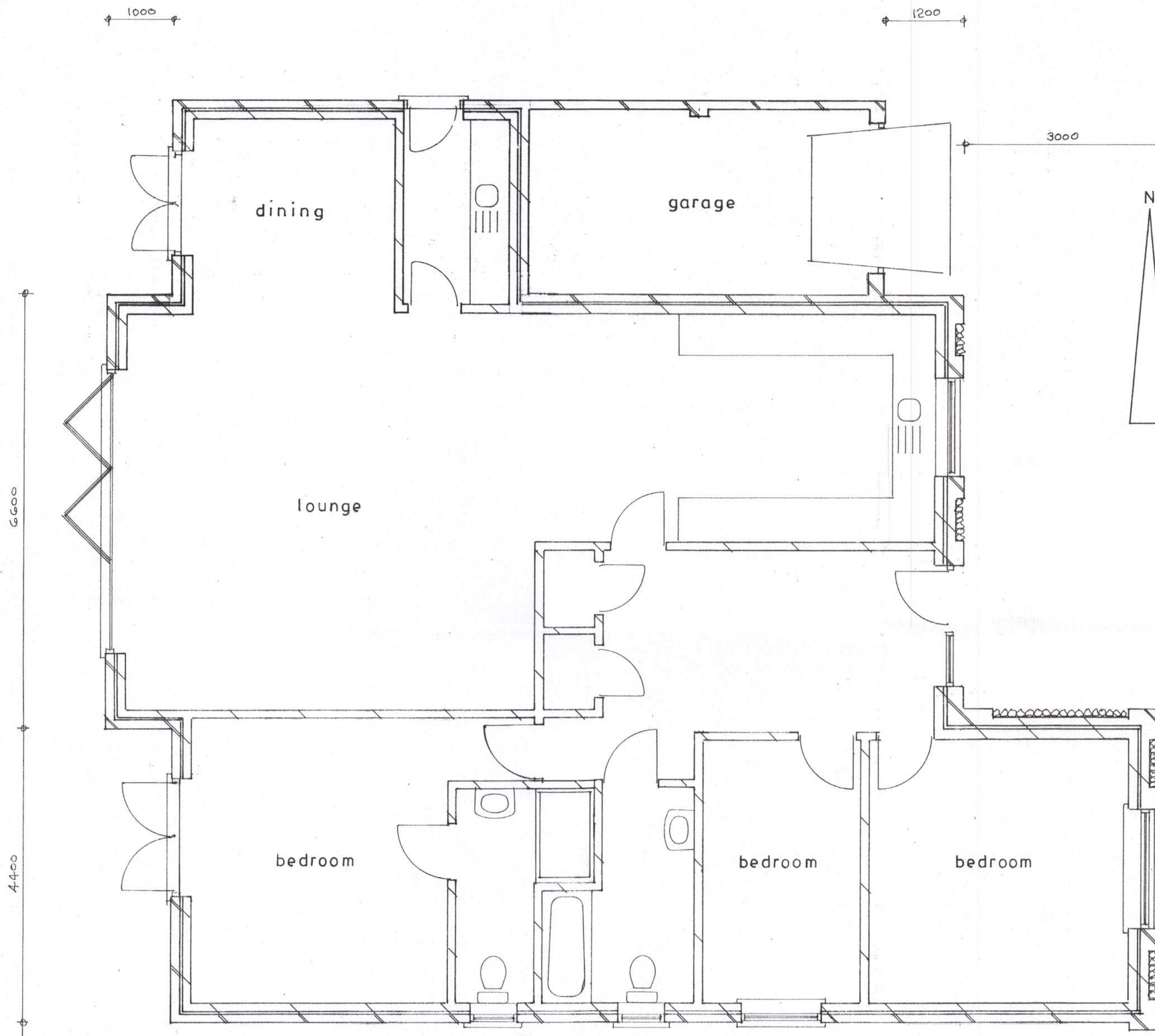
Plan 1 : 50
