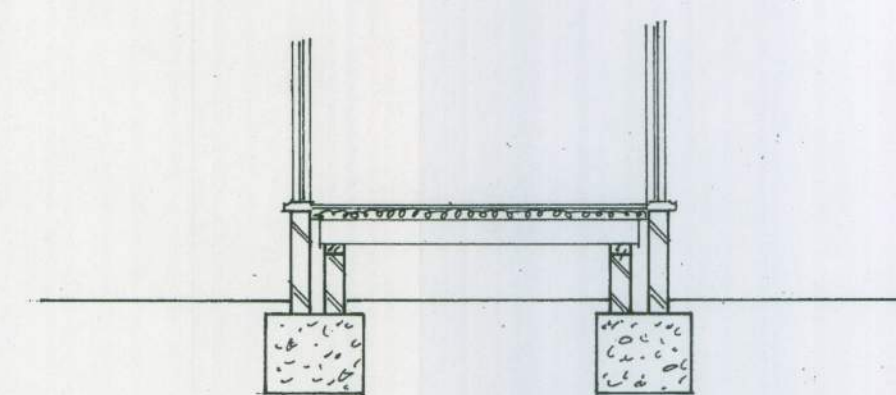
section 1 : 50
