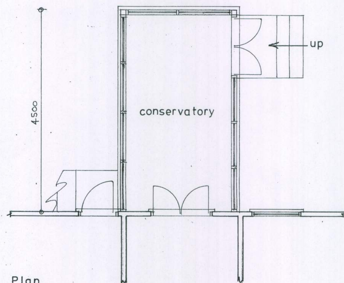
Plan 1 : 50
