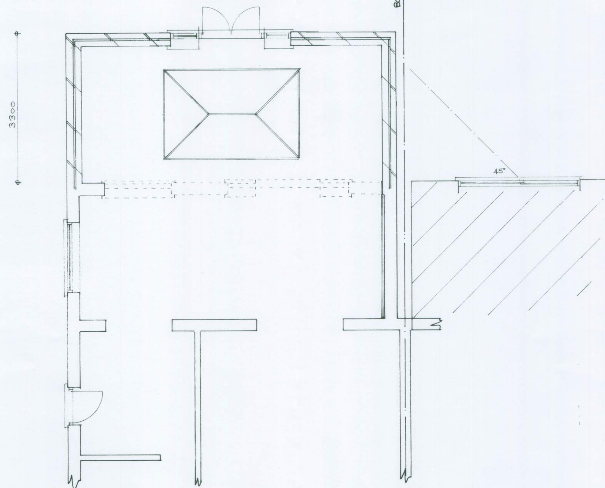
Plan 1 : 50
