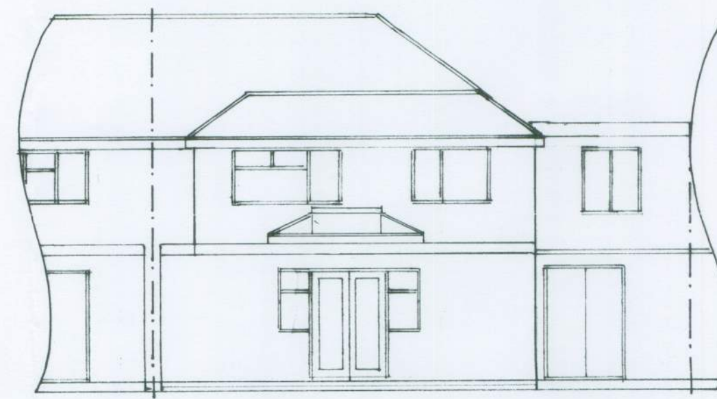
east 1 : 100
