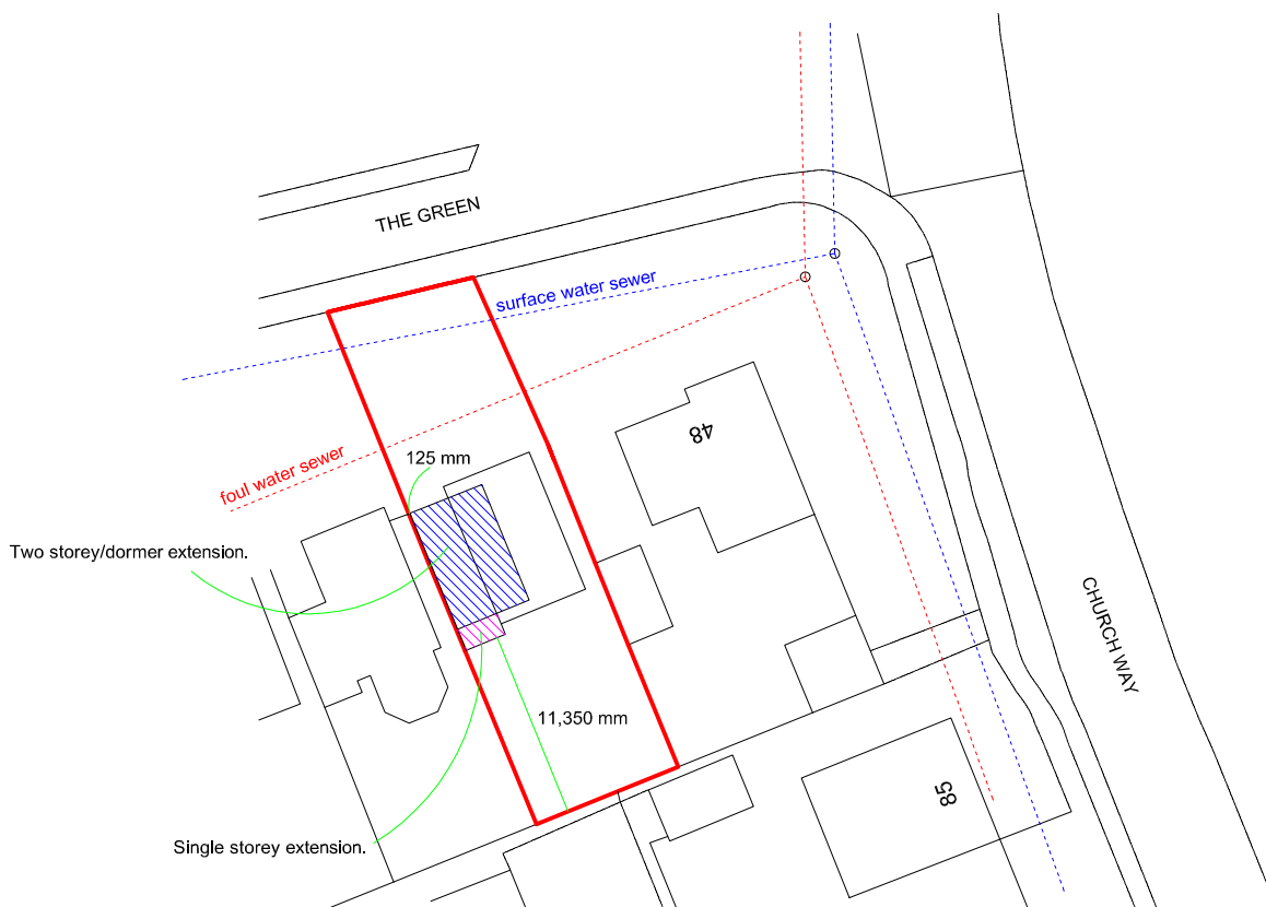
SITE PLAN - 1/500
