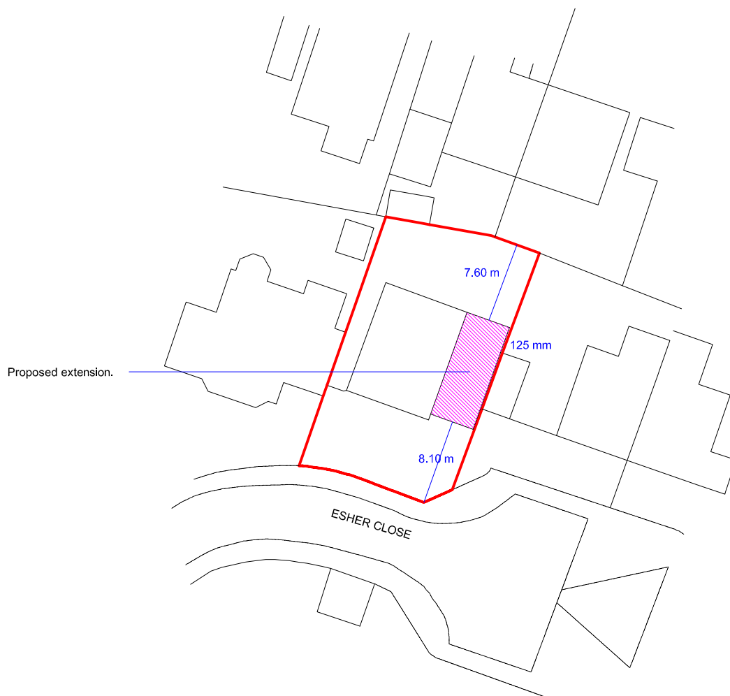
SITE PLAN - 1/500
