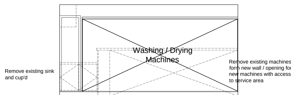
Elevation 3
