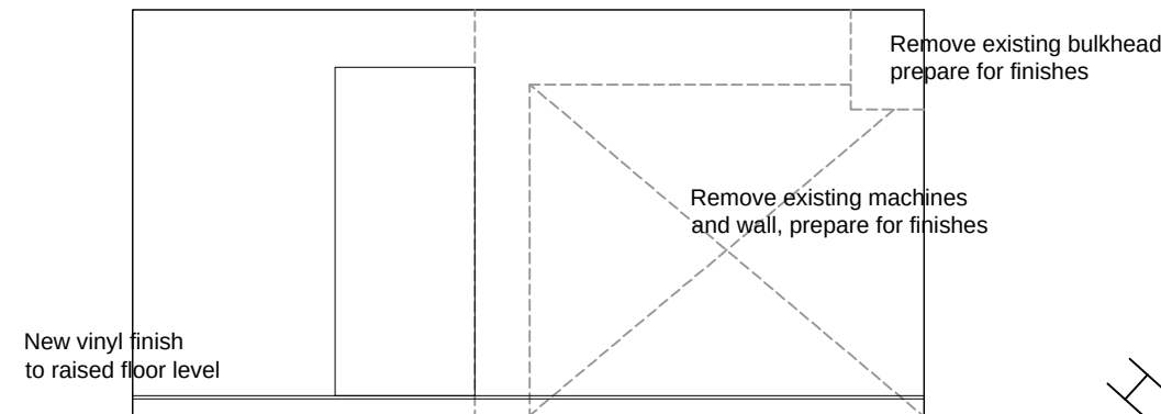
Elevation 5
