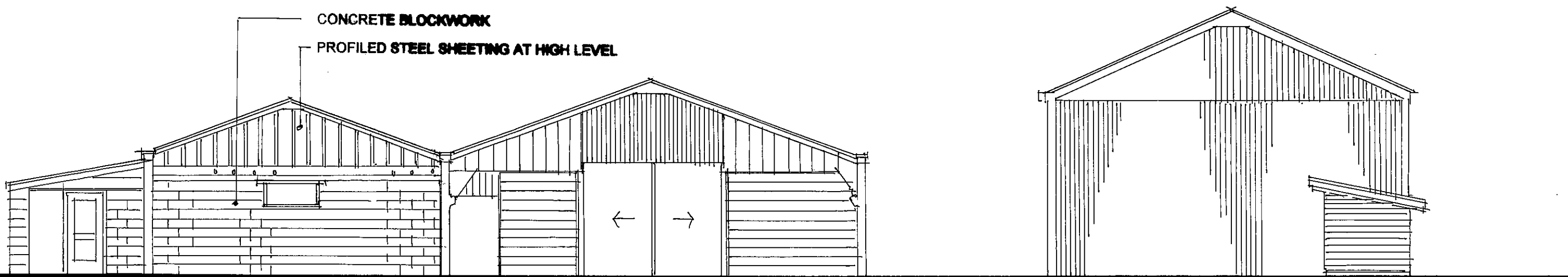
ELEVATION B
