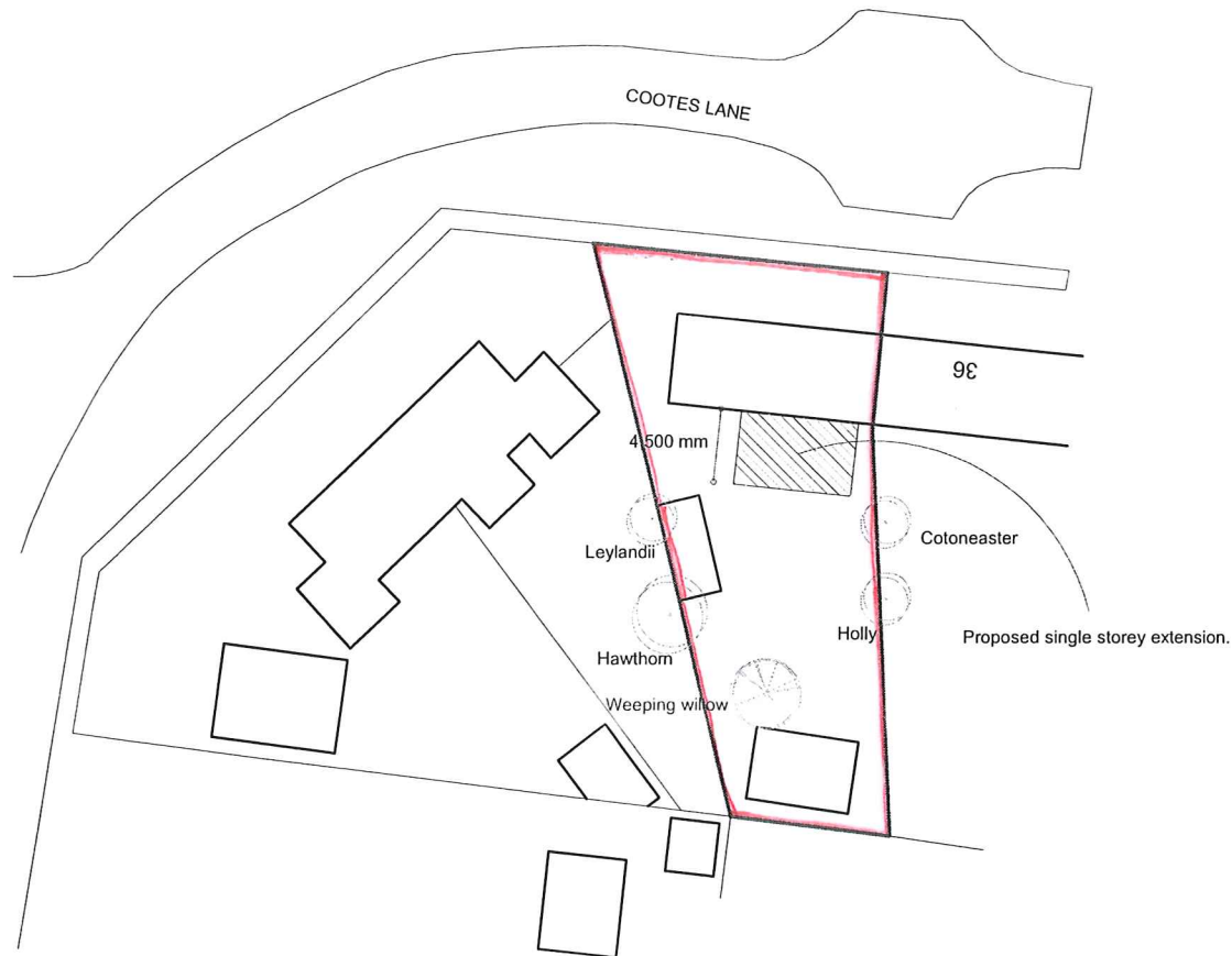
SITE PLAN - 1/500
