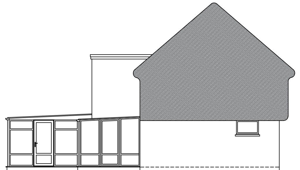
RIGHT ELEVATION
