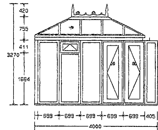
RIGHT ELEVATION
