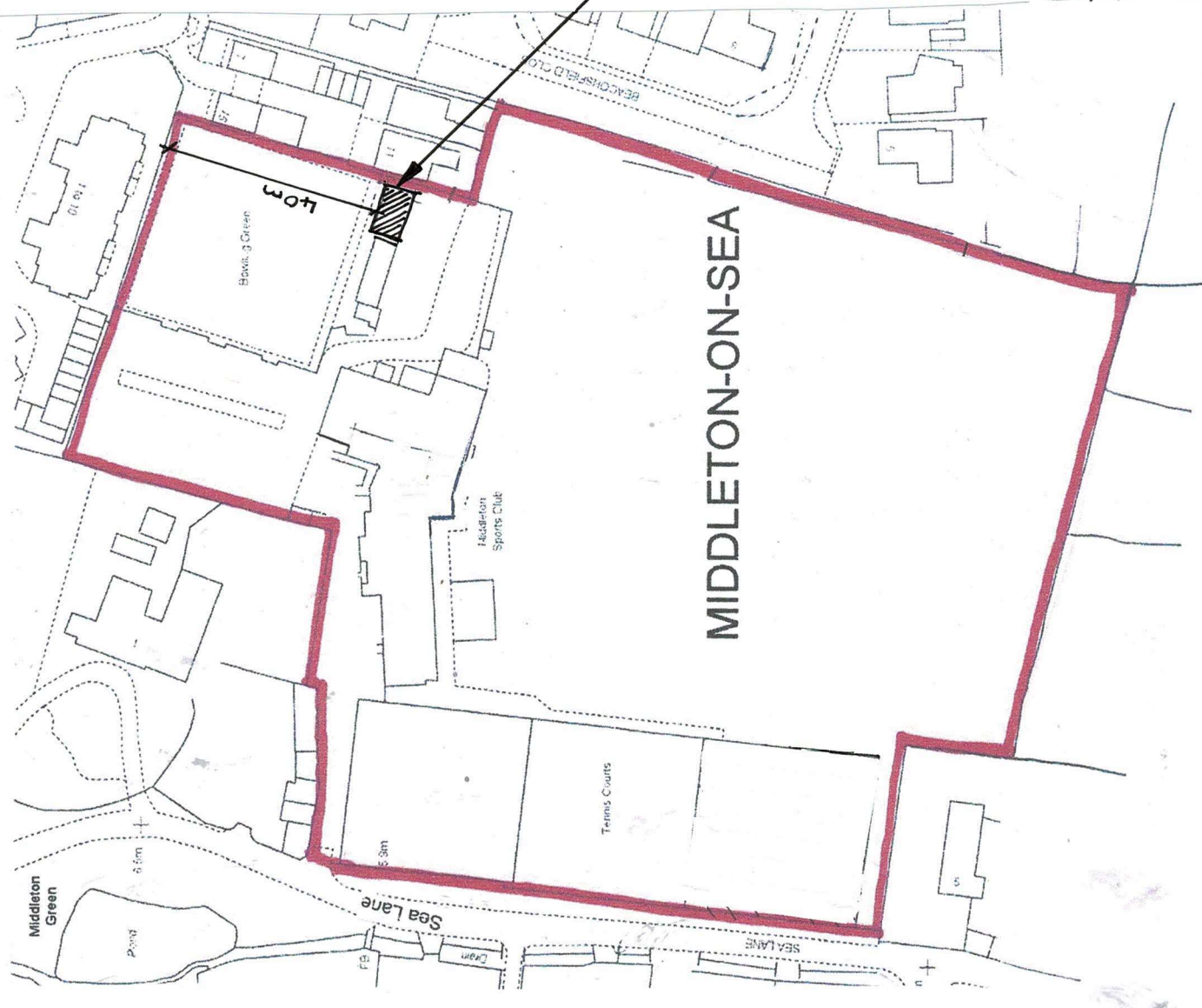
SITE PLAN 1:1250
