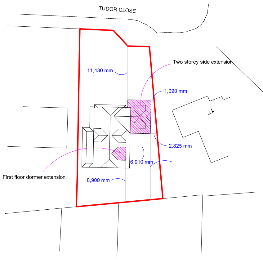
SITE PLAN - 1/500
