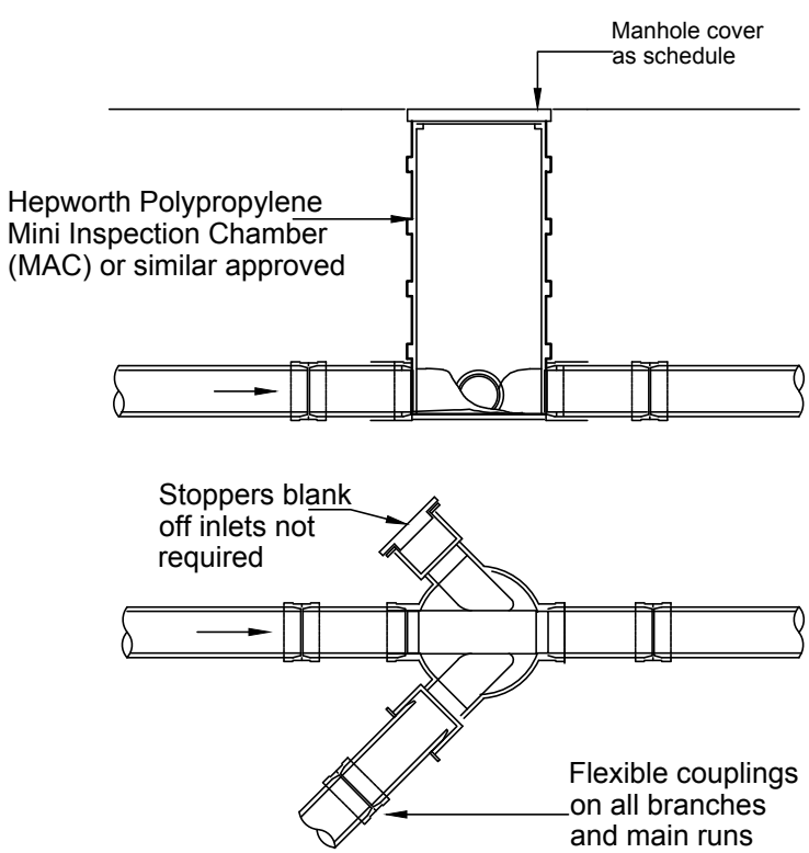
MINI ACCESS CHAMBER
