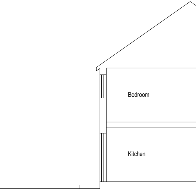
Existing Section A-A 1:100
