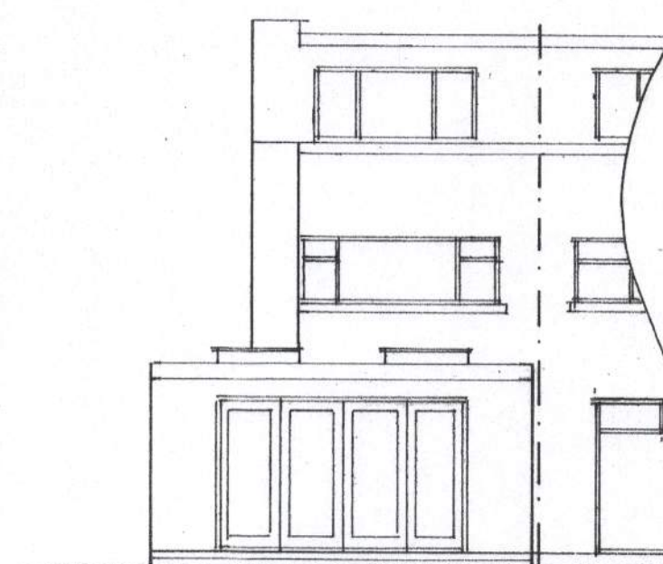
west 1 : 100
