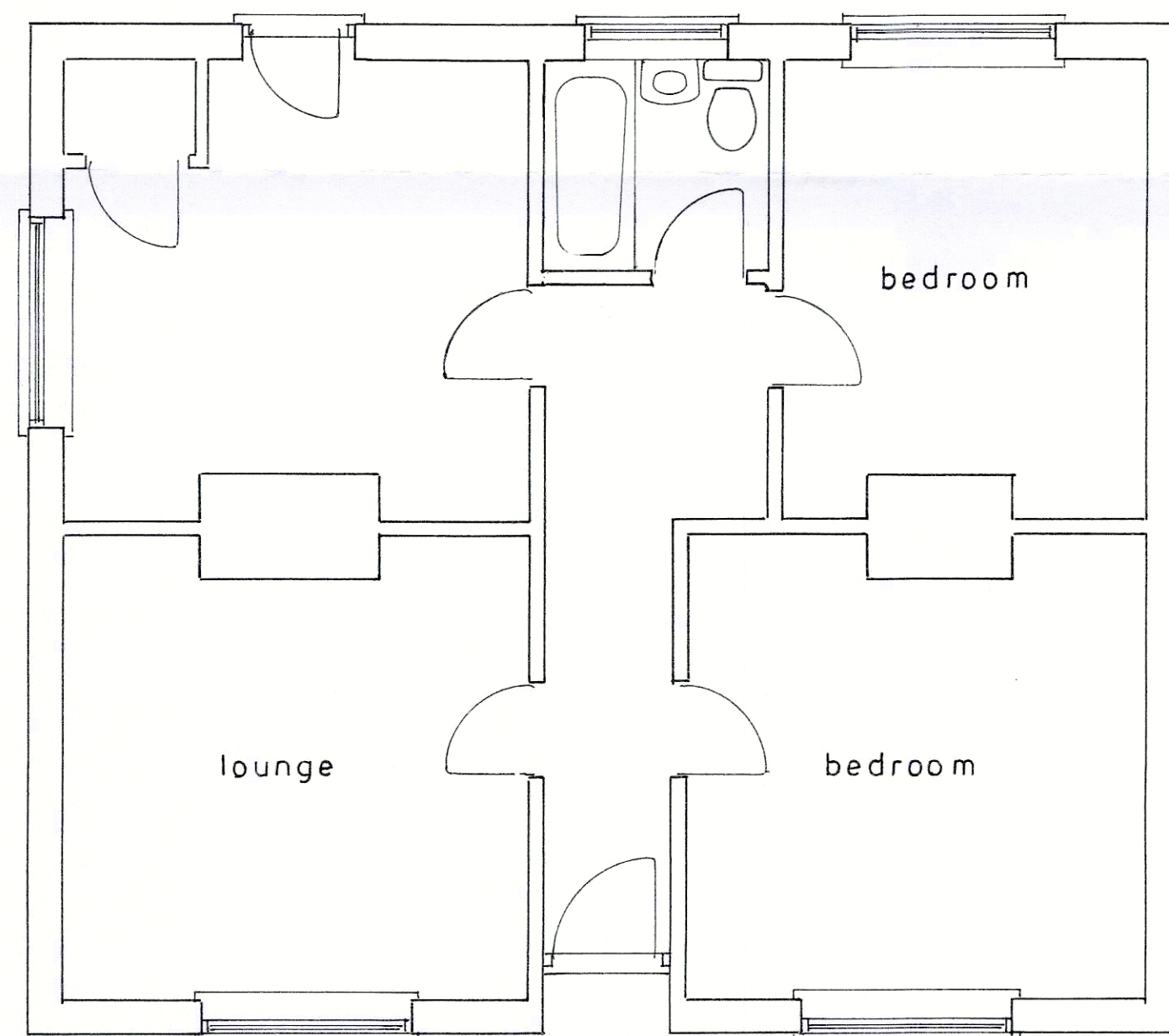
Plan 1 : 50
