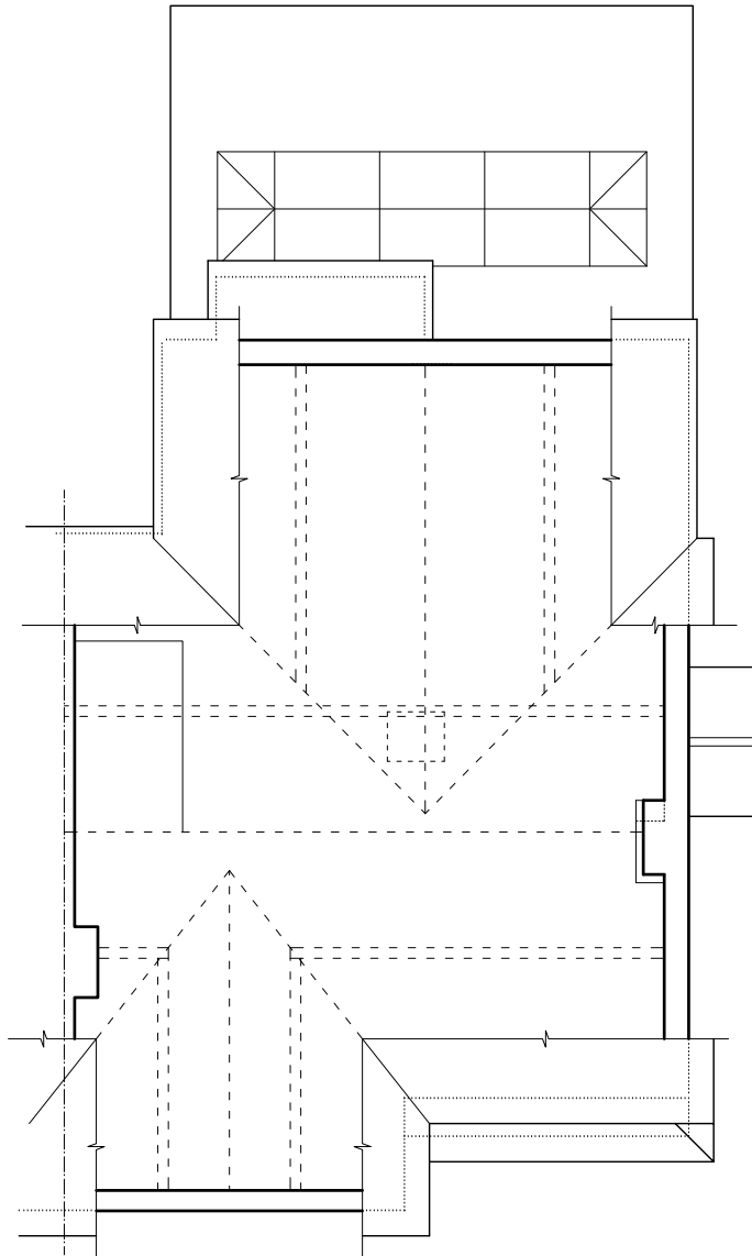
Loft Plan
