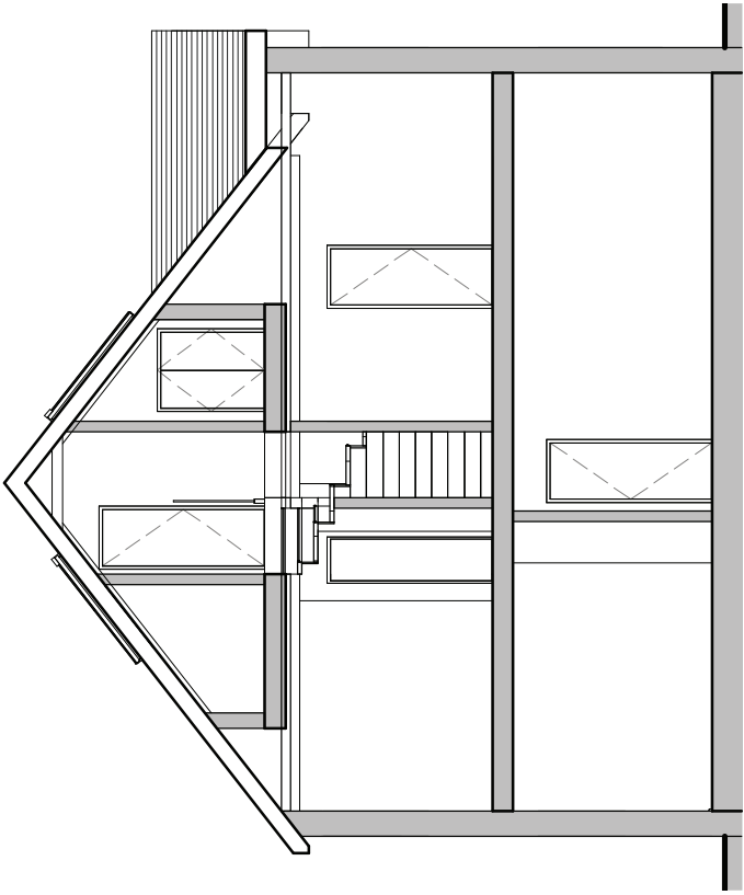
Section 1 1 : 100
