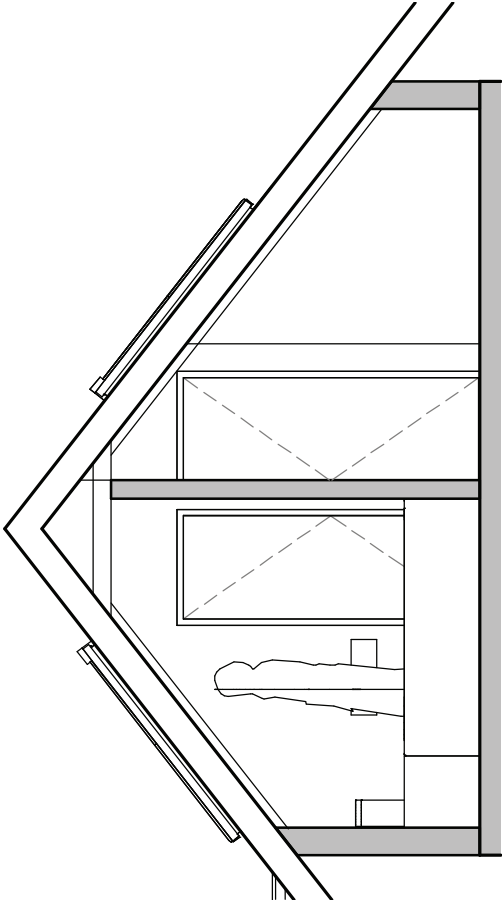
Section 3 1 : 50
