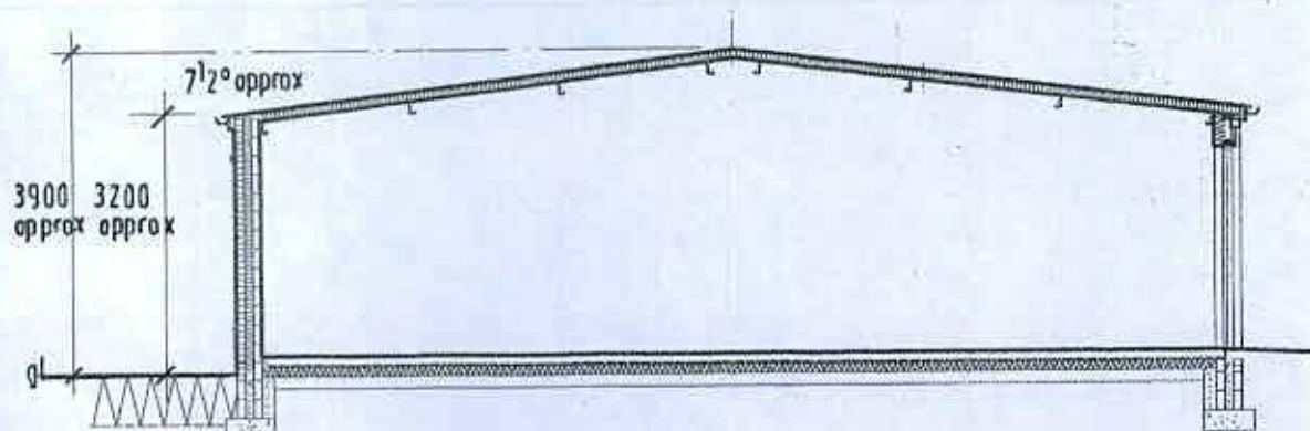
SECTION A:A 1/100
