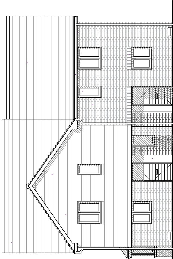
04 Elevation 01 2100 Scale: 1:100
