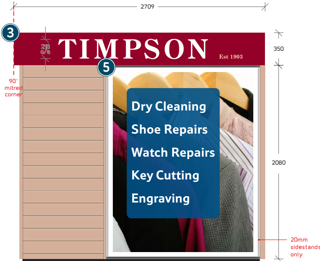
Right elevation
