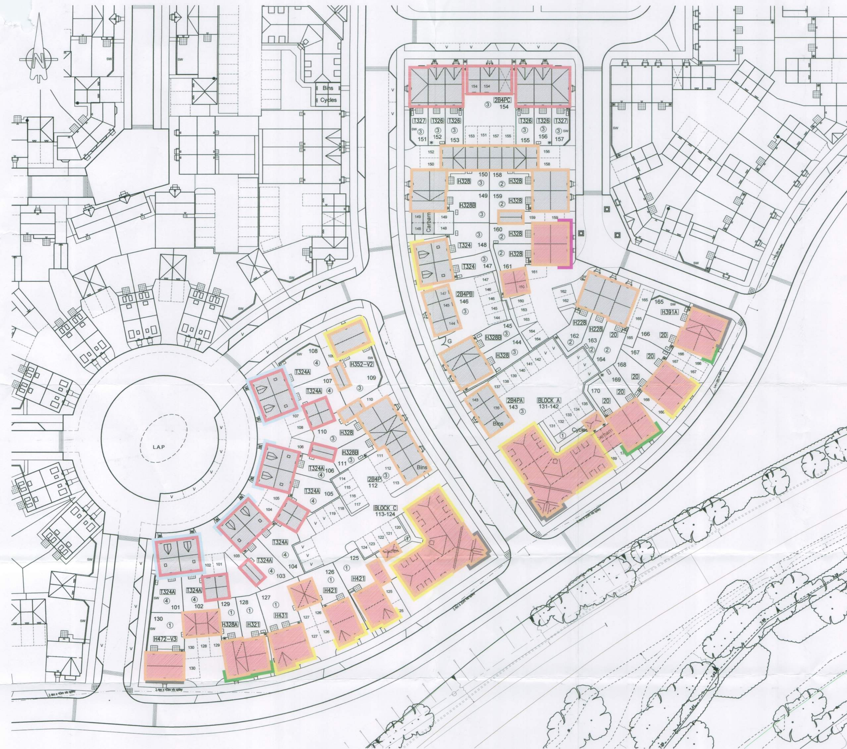
SITE LAYOUT 1:500
