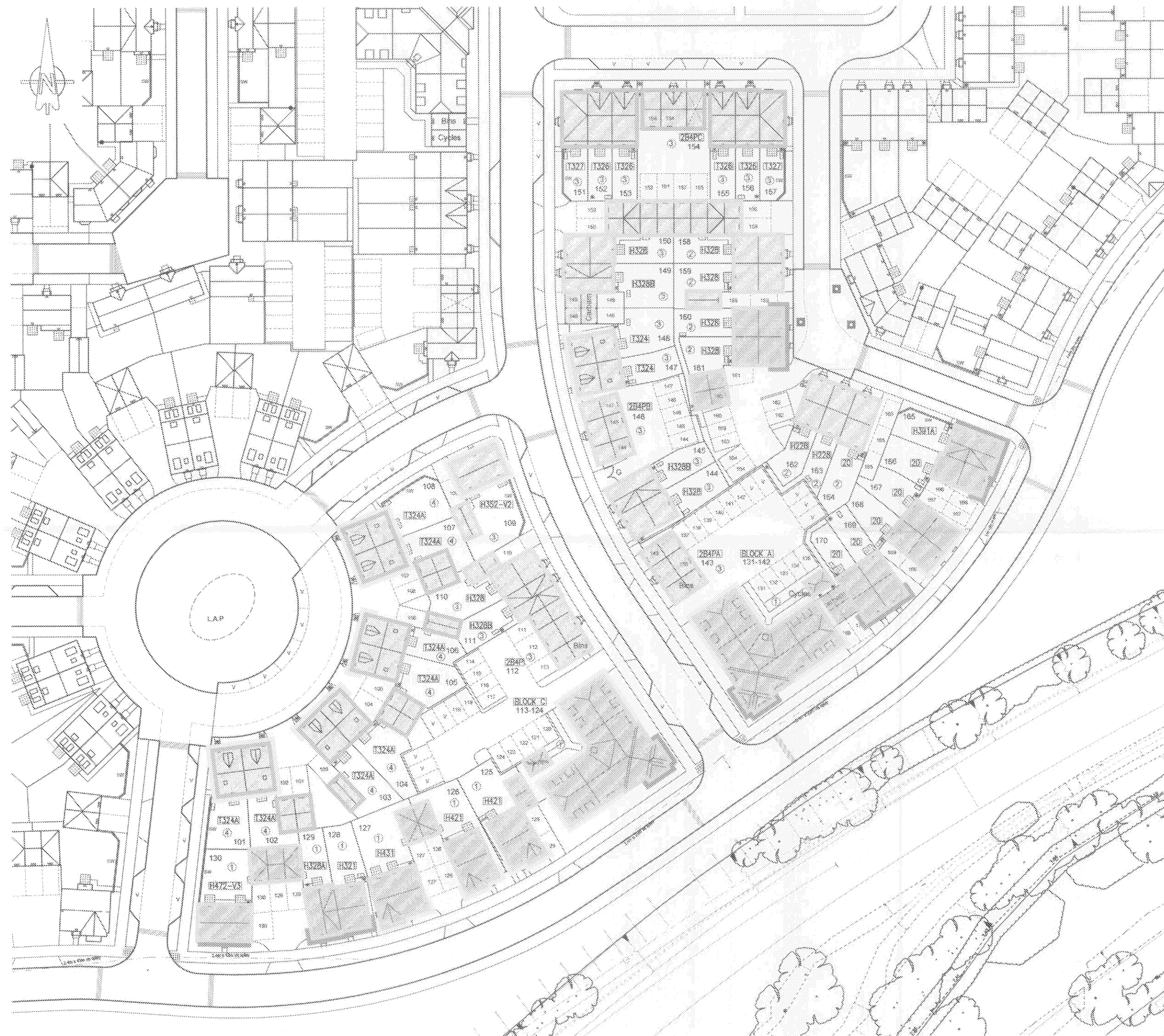
SITE LAYOUT 1:500
